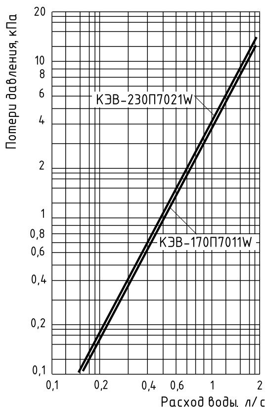
Рисунок 1. Гидравлические характеристики
