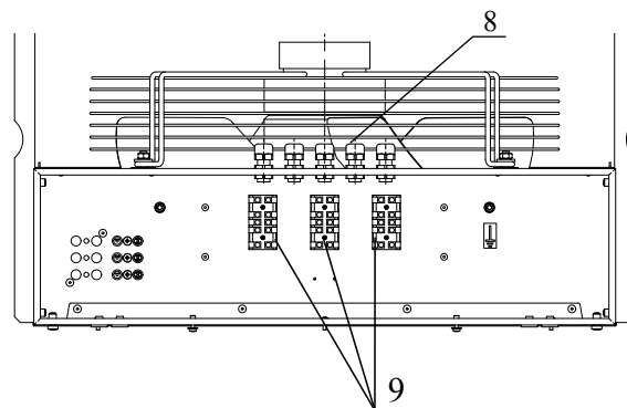
Вид А
