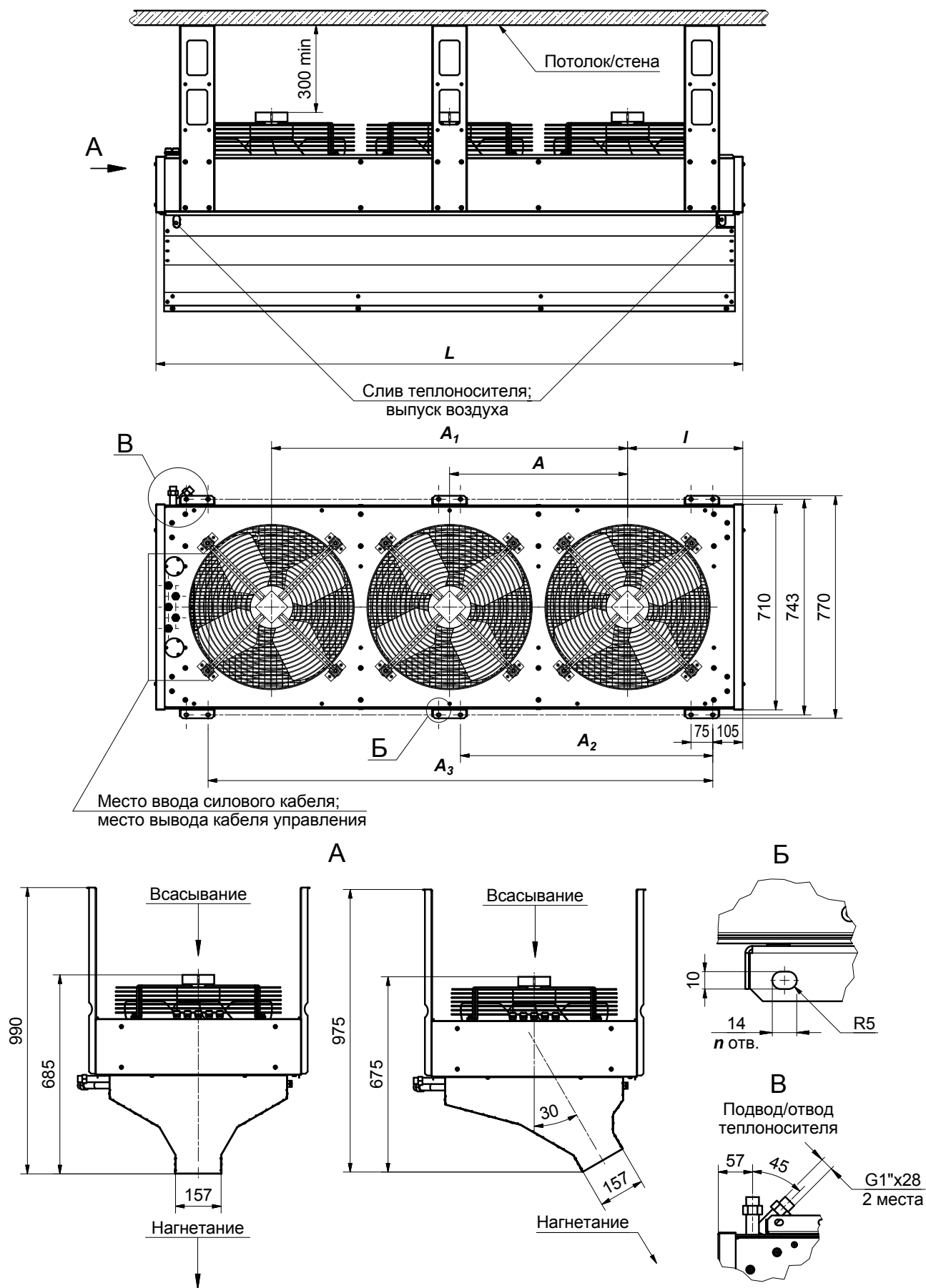
Рисунок 6. Габаритные и присоединительные размеры
