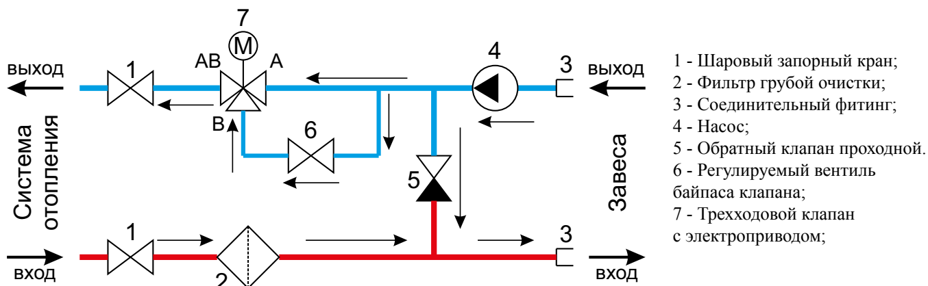
Рисунок 4. Схема узла терморегулирования с трехходовым регулирующим клапаном и насосом.
