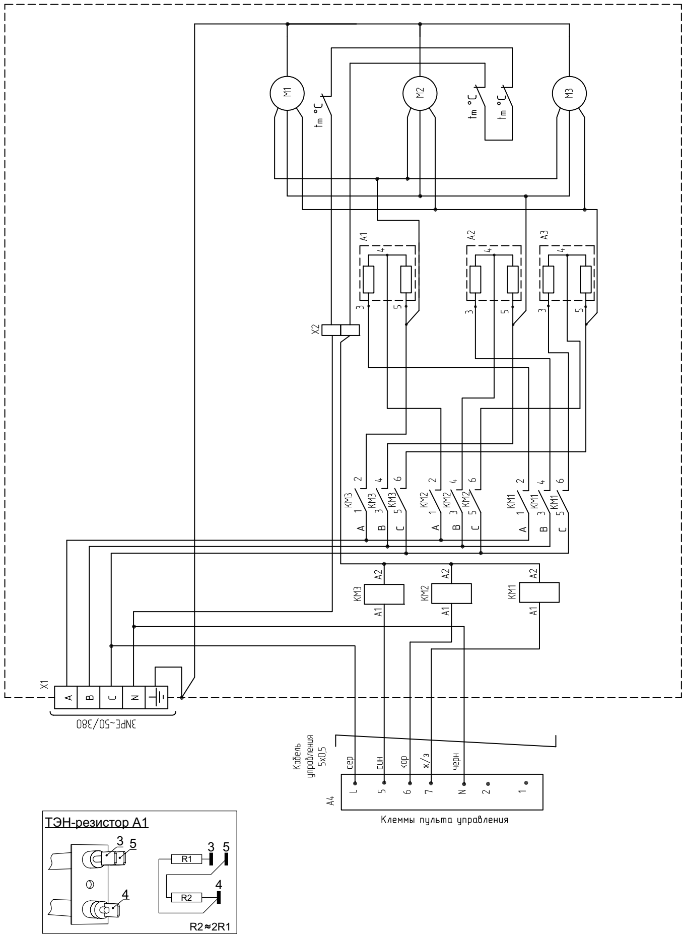
Рисунок 13. Электрическая схема занавесы КЭВ-230П7020W
