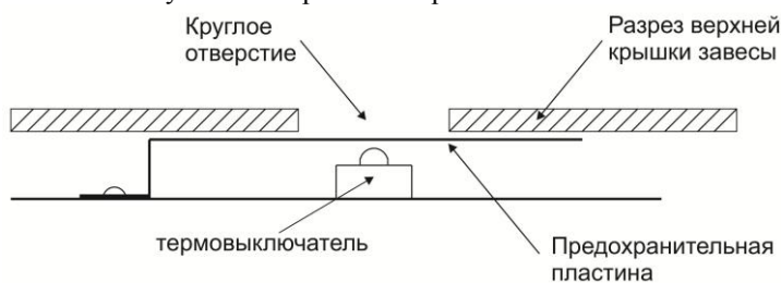
Рисунок 4-Аварийный термовыключатель
