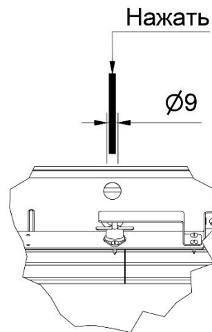
Рисунок 4-Аварийный термовыключатель
