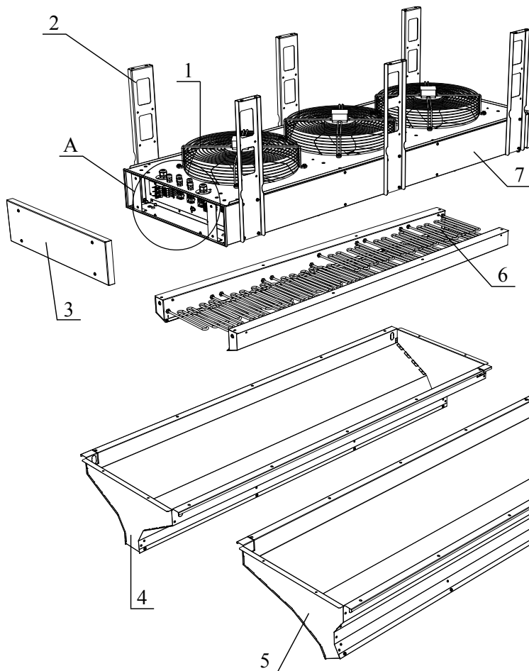
Рисунок 1. Воздушно-тепловая завеса
