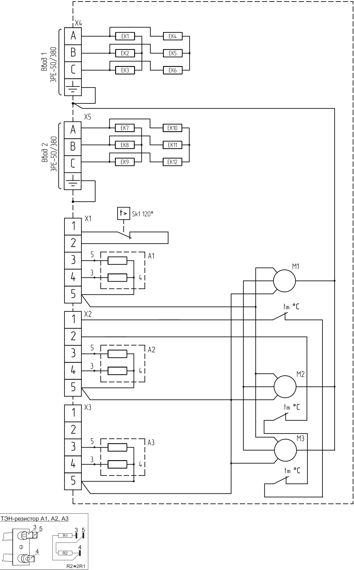
Рисунок 5. Электрическая схема завесы КЭВ-24П5061Е, КЭВ-36П5061Е
