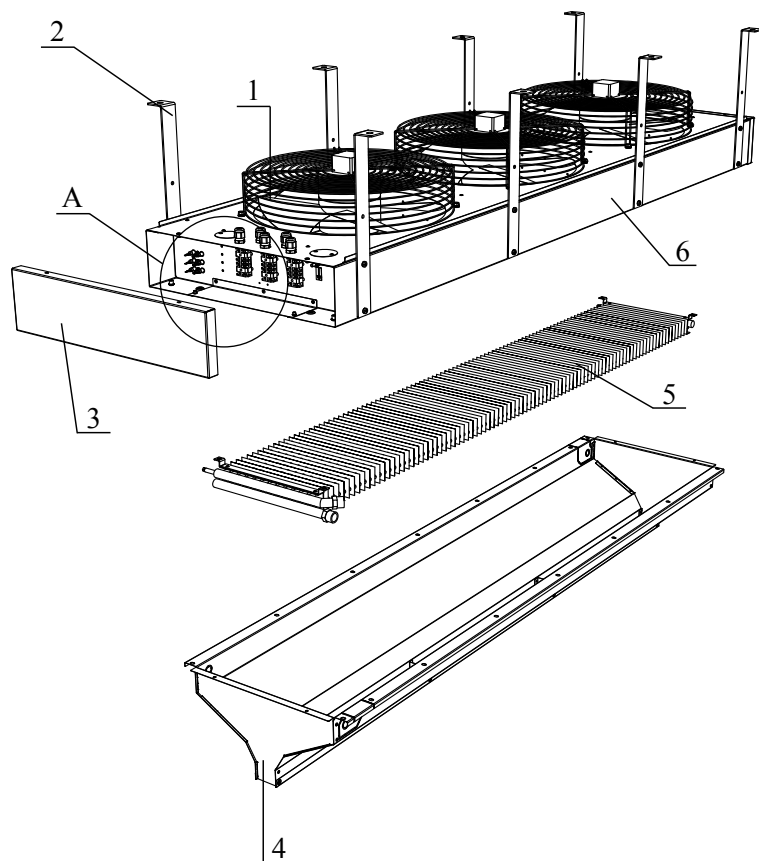
Рисунок 2. Воздушно-тепловая завеса
