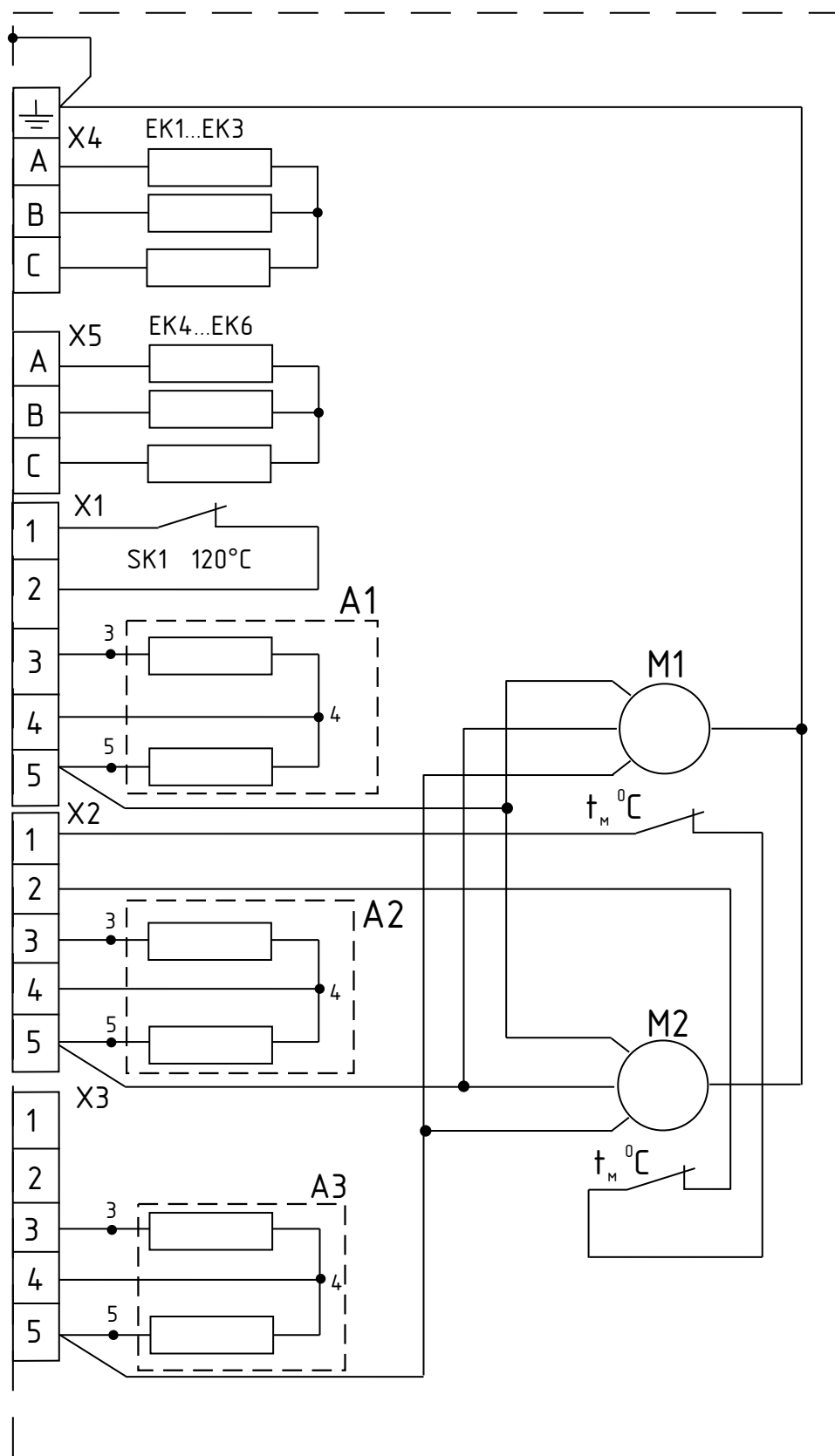
Рисунок 3. Электрическая схема занавесы КЭВ-12П4050Е, КЭВ-18П4050Е
