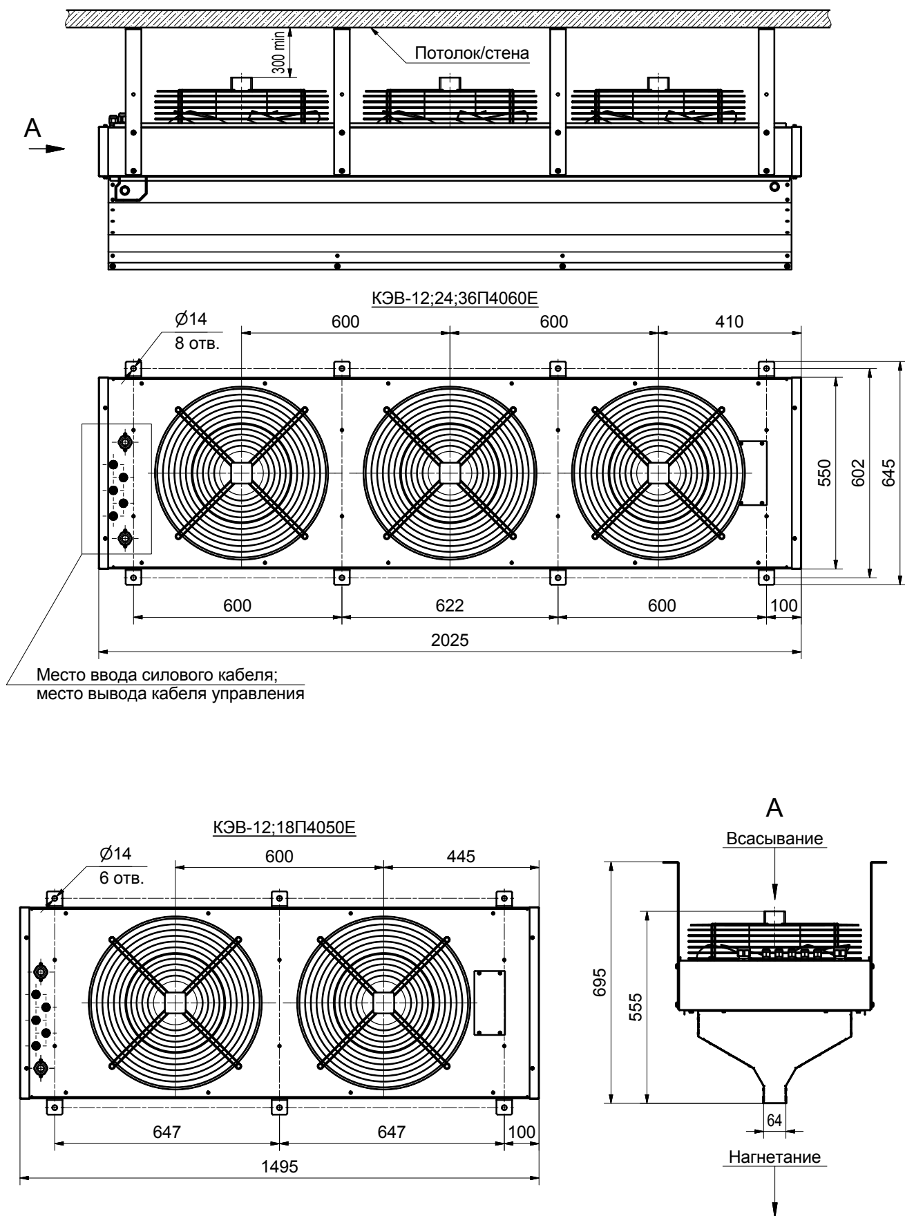
Рисунок 2. Габаритные и присоединительные размеры
