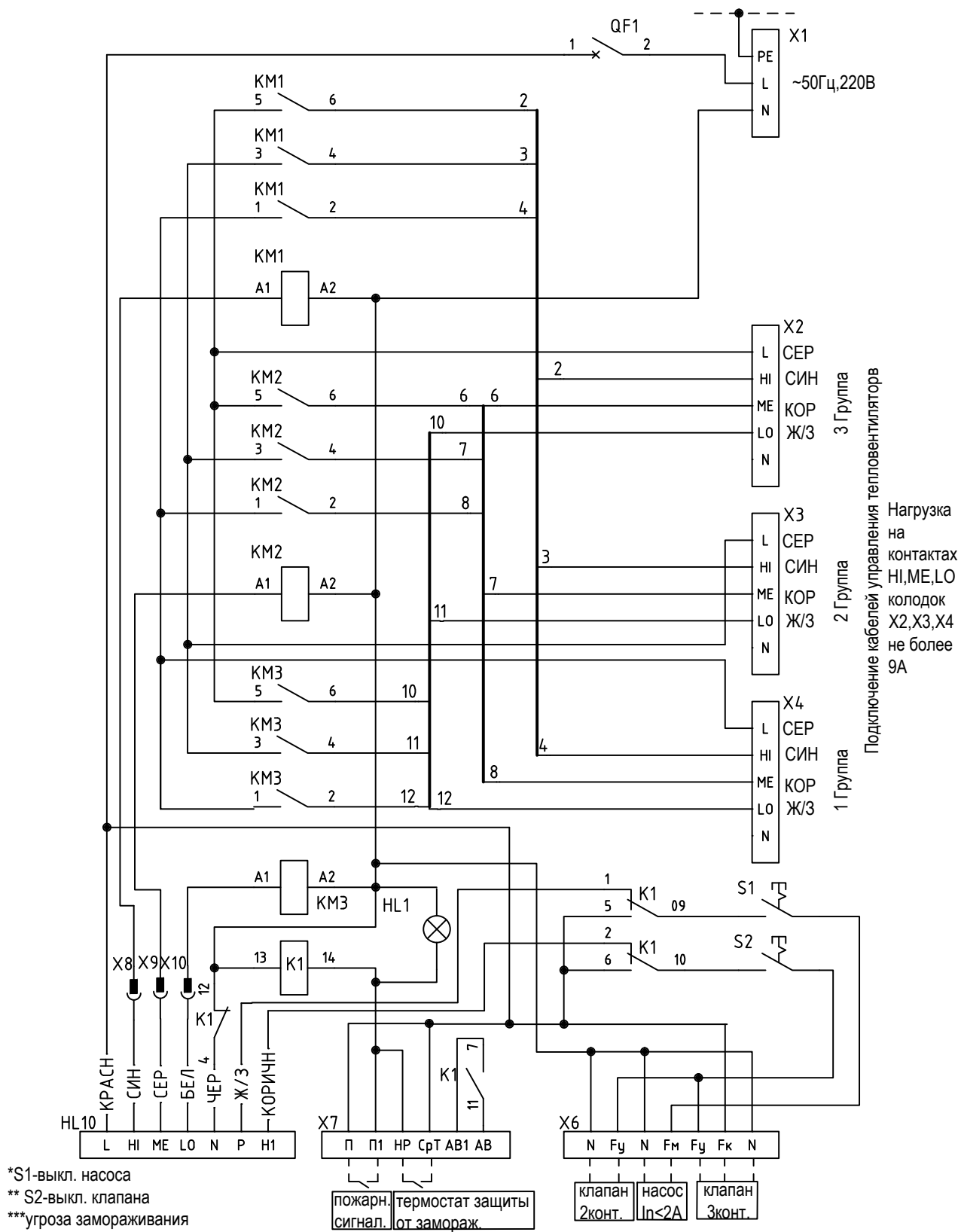
Рисунок 1. Электрическая схема ПКУ-W1
