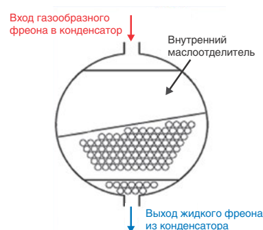
Встроенный одноступенчатый маслоотделитель конденсатора
