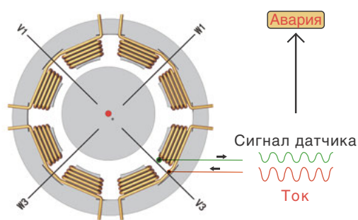
Схема управления подшипником
