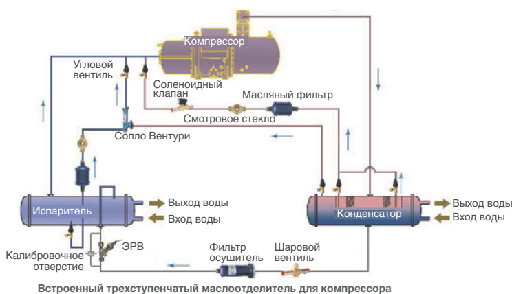
Встроенный трехступенчатый маслоотделитель для компрессора
