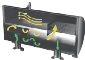
Экономайзер
