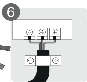
Подключите провода
