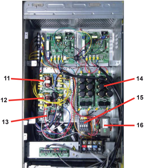
Щит управления Нижняя часть (расположена под верхней частью, верхняя часть поворачивается на петлях)
