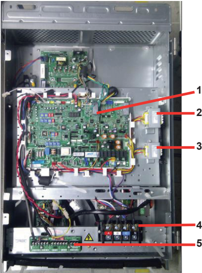
Щит управления Верхняя часть
