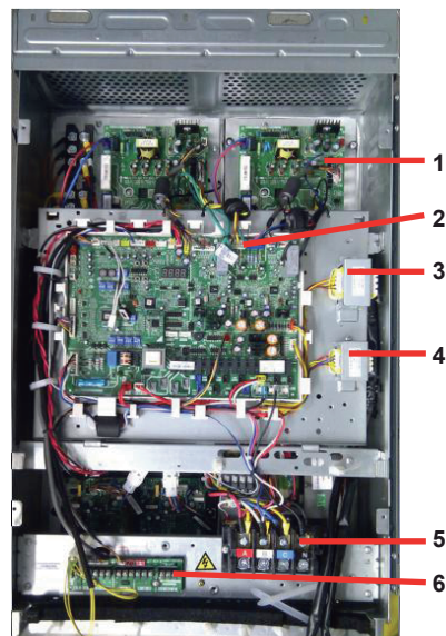
Щит управления Верхняя часть
