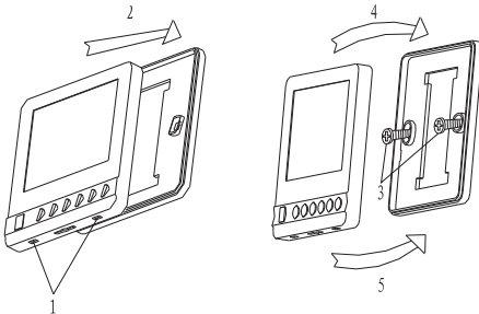
Установка проводного пульта управления
