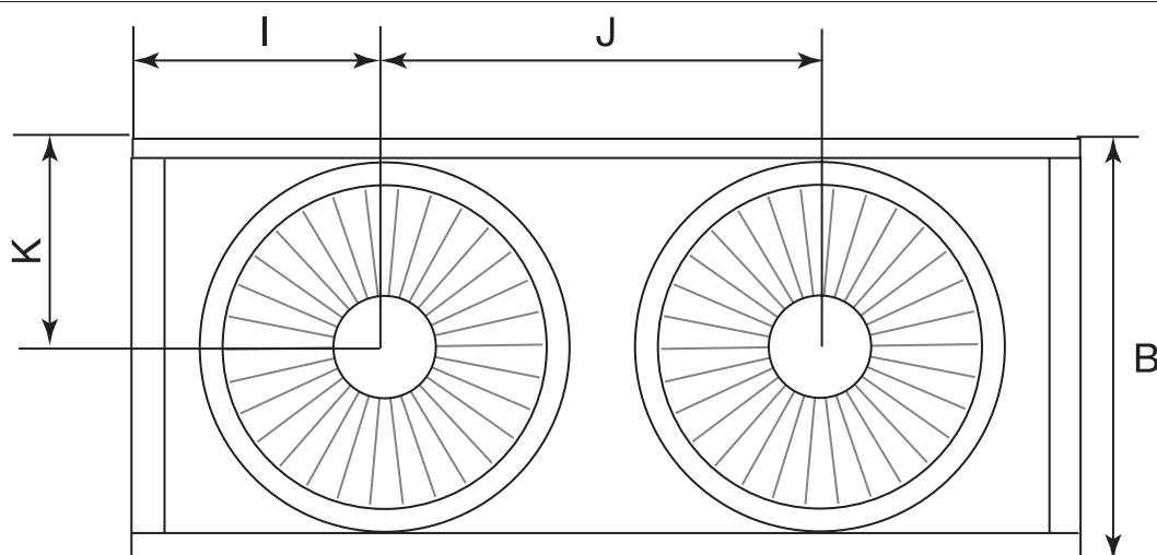
Вид сверху
