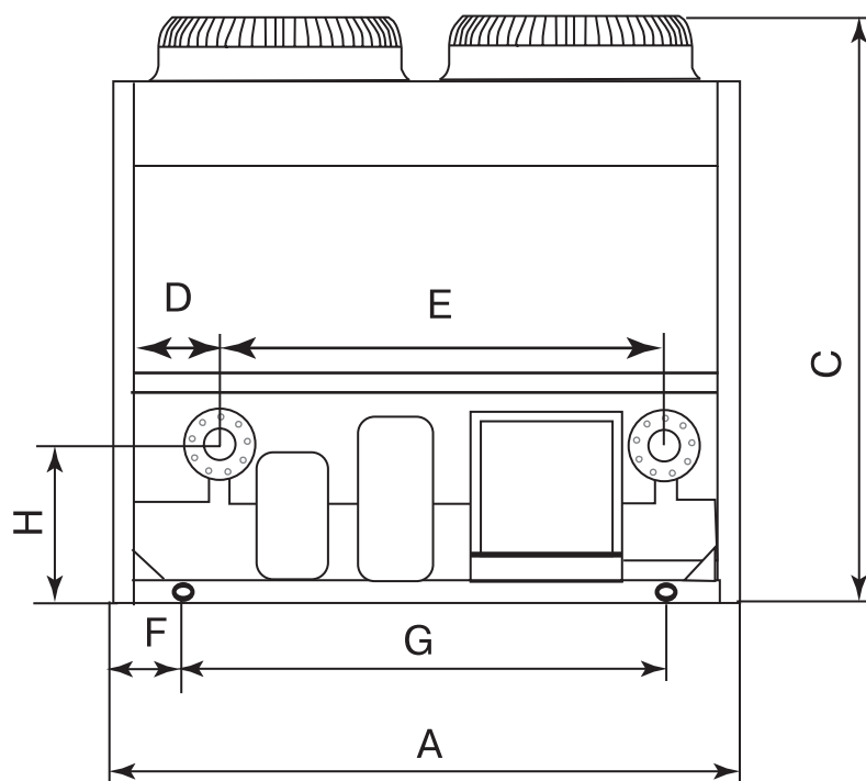
Вид спереди
