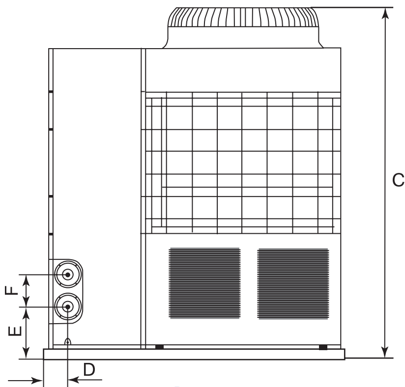
Вид спереди
