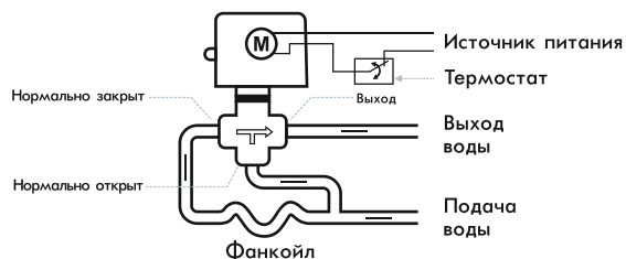
Рис. 4. 3-ходовой клапан
