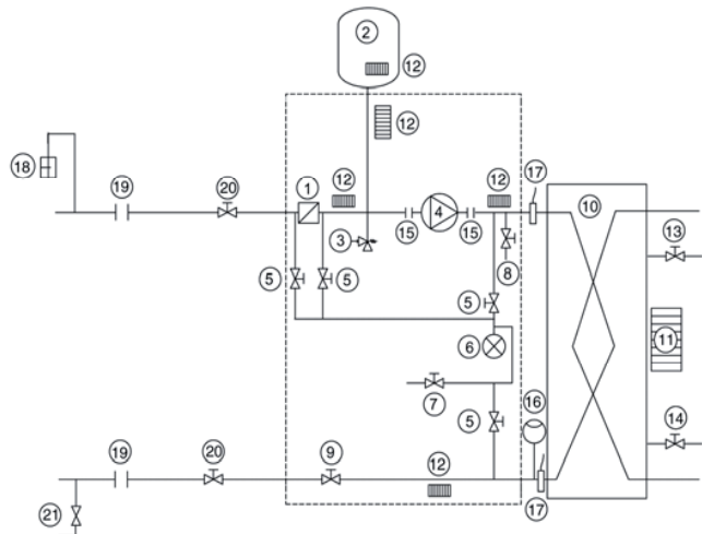
Типовая схема гидро модуля
