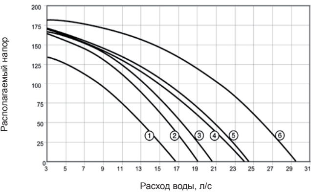
Насос низкого давления (опция гидронного модуля)
