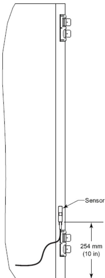
Рис. 33 – Расположение датчиков Motormaster, модель 38AUD*12-14
