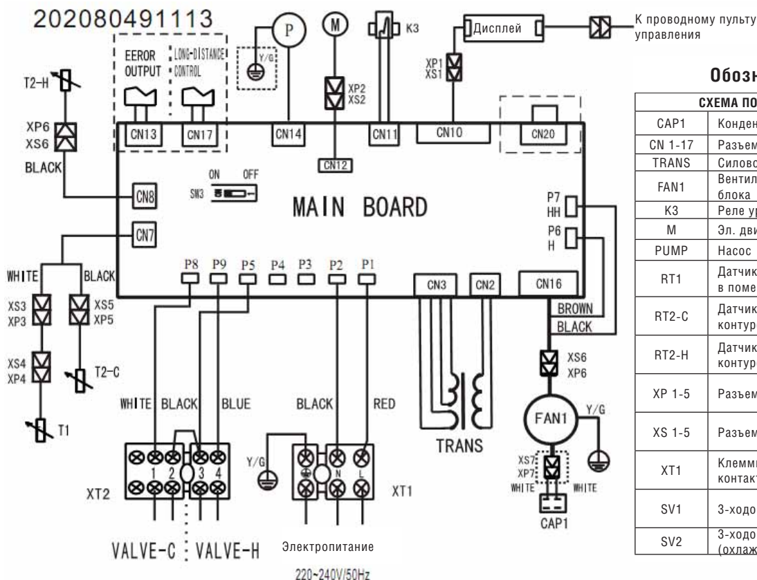
Рис. №4. Электрическая схема ACF-50CS/4
