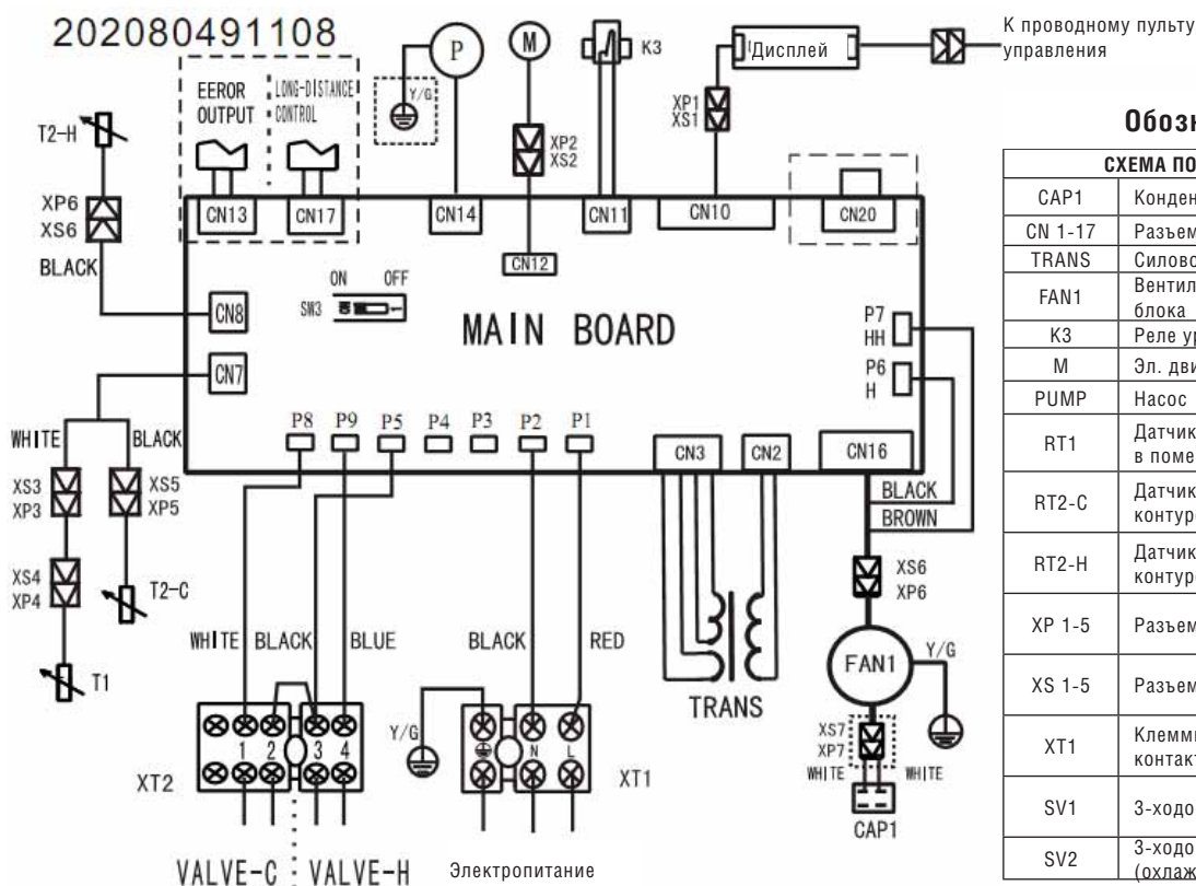
Рис. №4. Электрическая схема ACF-50CS/4
