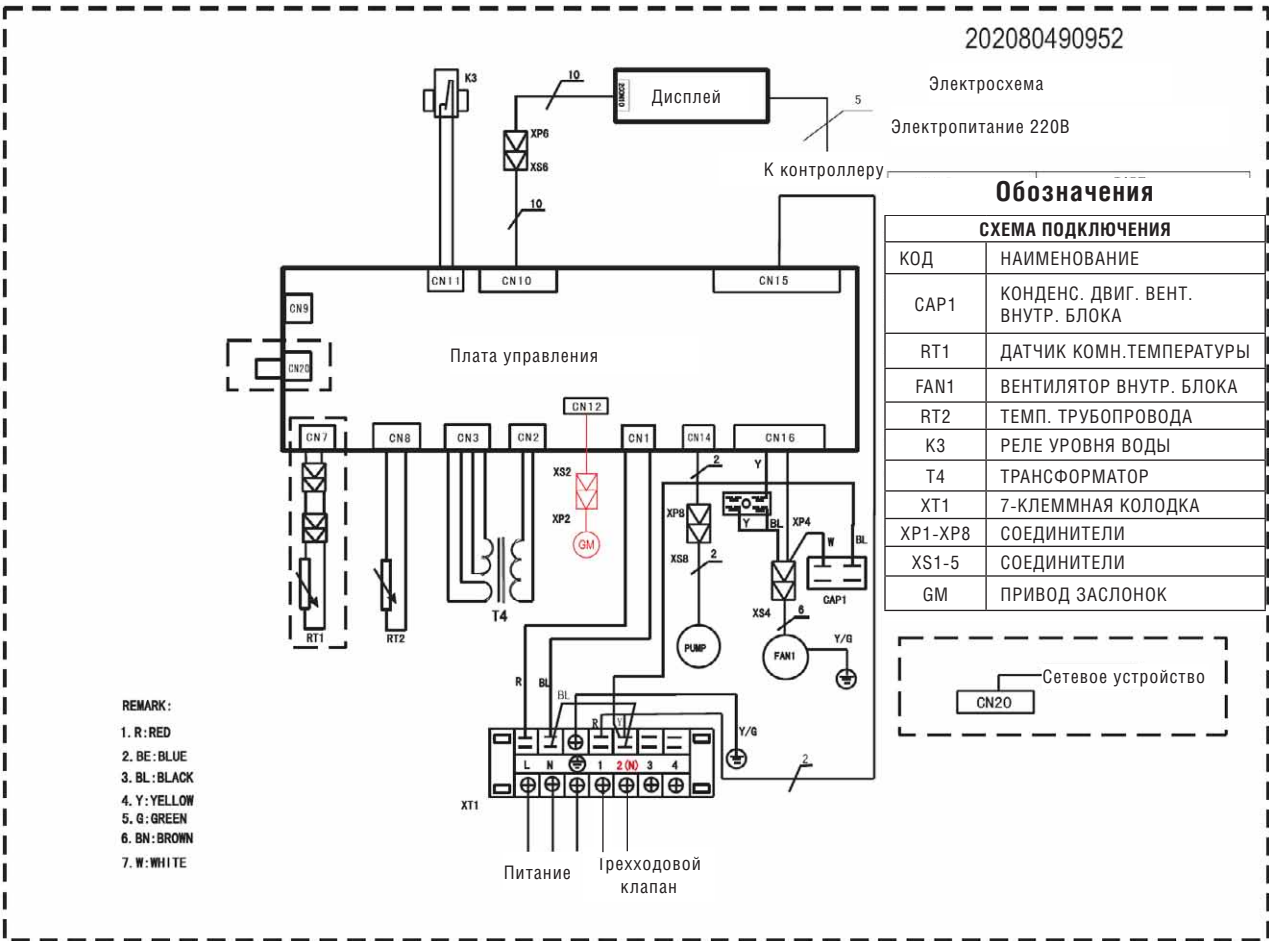
Рис. №4. Электрическая схема ACF-CS.
