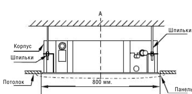
Рис. №8. Установка фанкойла.
